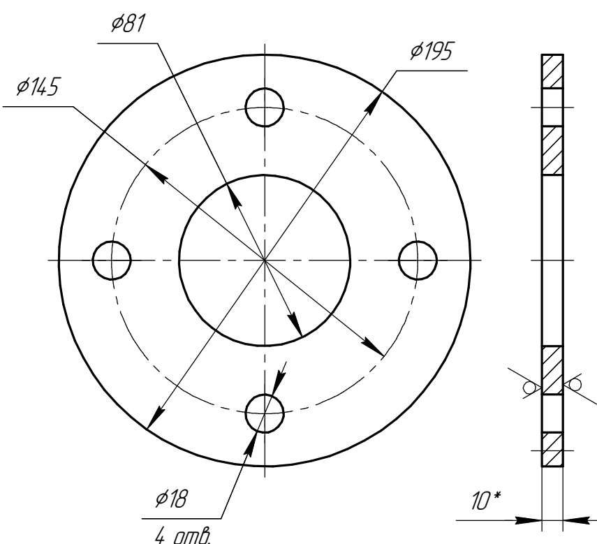
Дет. поз. 2 (1:2,5)
