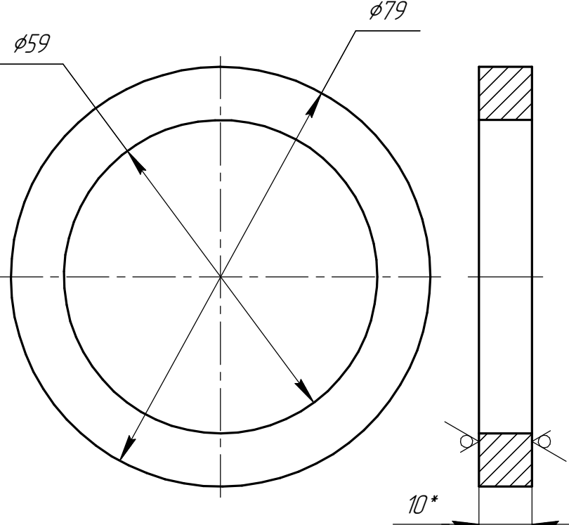
Дет. поз. 3 (1:1)
