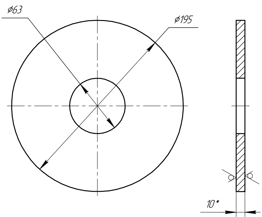
Дет. поз. 1 (1:2,5)
