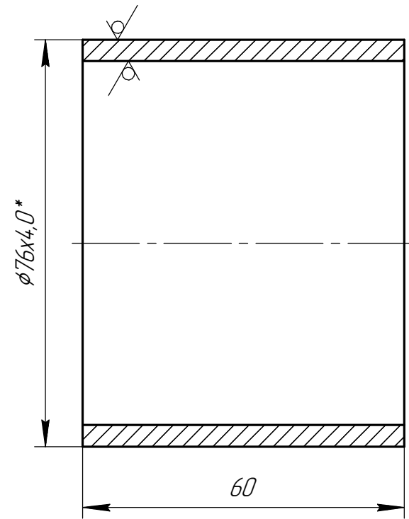
Дет. поз. 5 (1:1)
